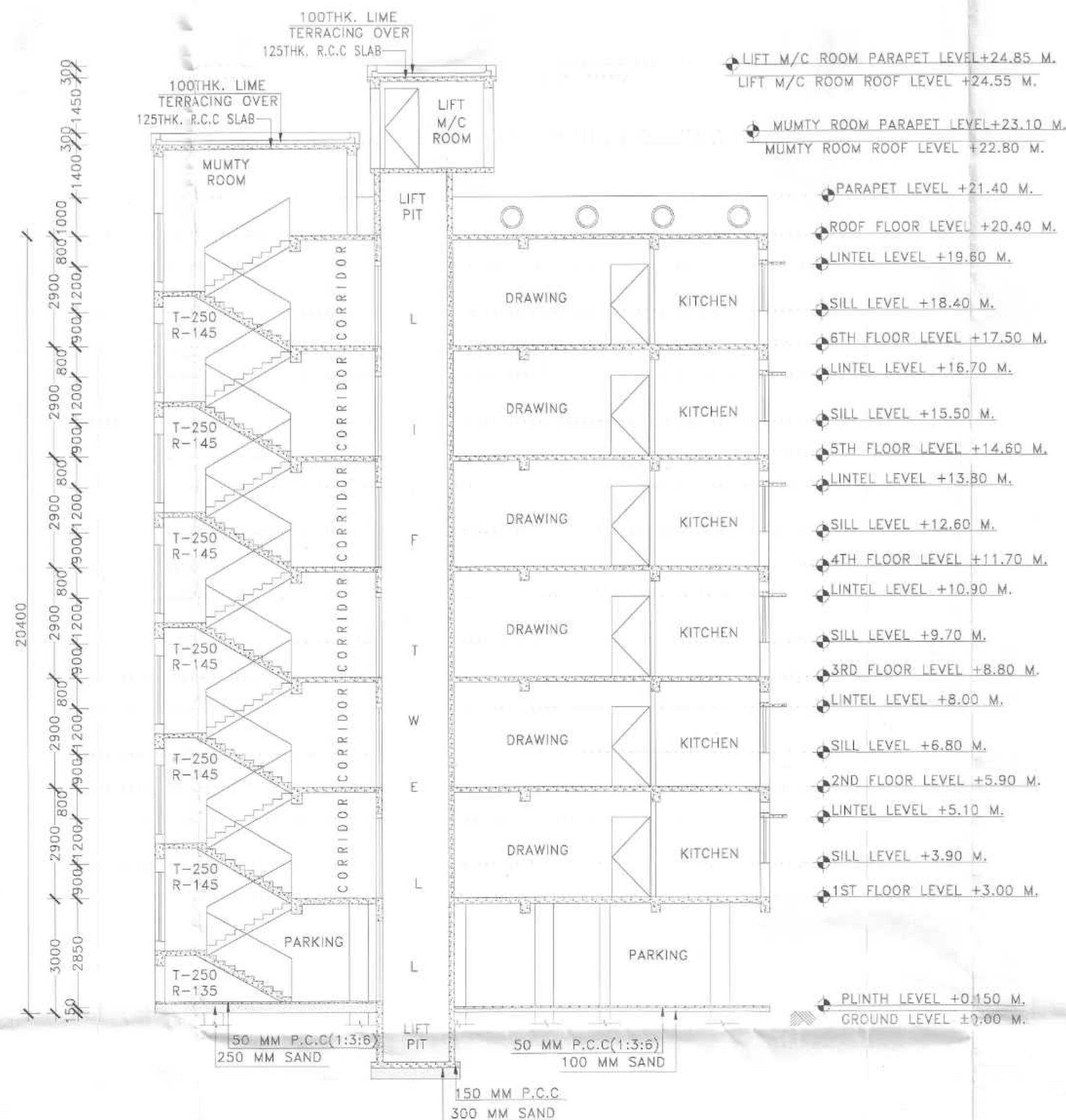
SECTION: -X-X SCALE: 1:100
