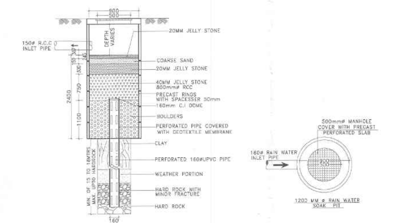
(D) SECTIONAL DETAILS OF RAIN WATER SOAK PIT SCALE: N.T.S.
