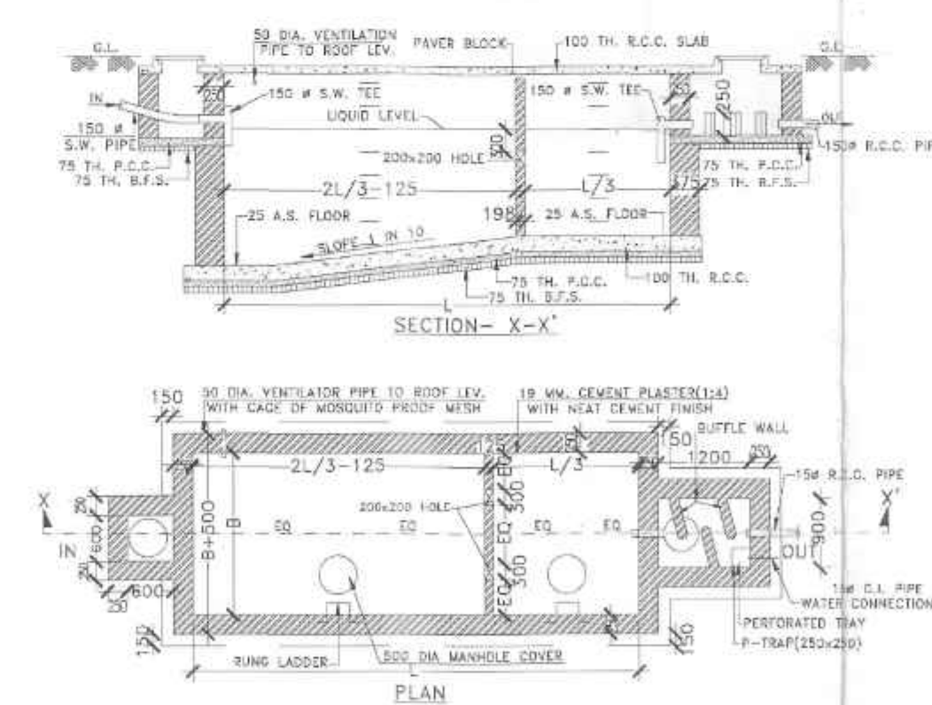
E DETAILS OF SEPTIC TANK SCALE: N.T.S.
